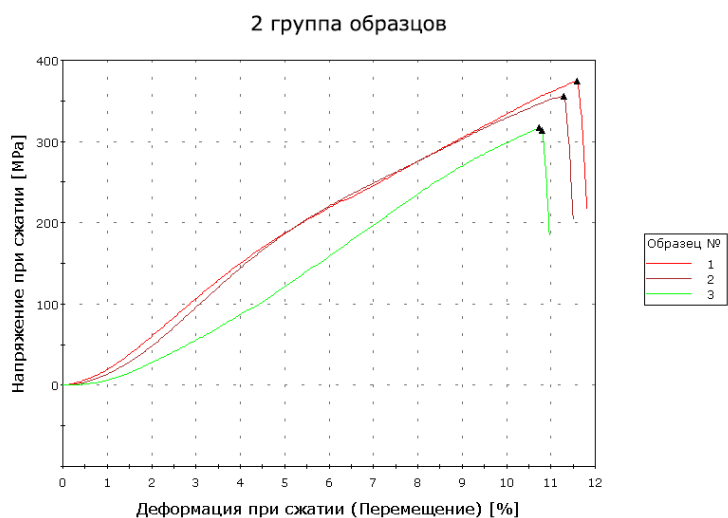
Рисунок 2 - Деформационные кривые при сжатии образцов 2 группы
