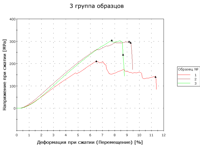
Рисунок 3 - Деформационные кривые при сжатии образцов 3 группы
