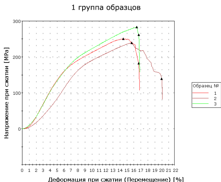
Рисунок 1 - Деформационные кривые при сжатии образцов 1 группы
